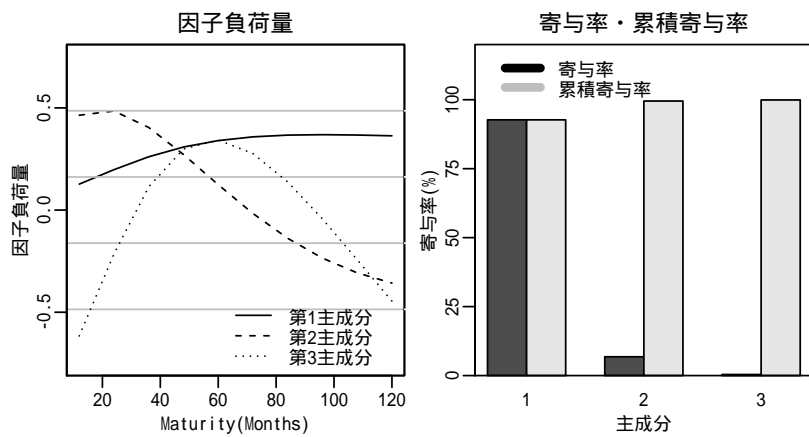
図1: PCA 結果
