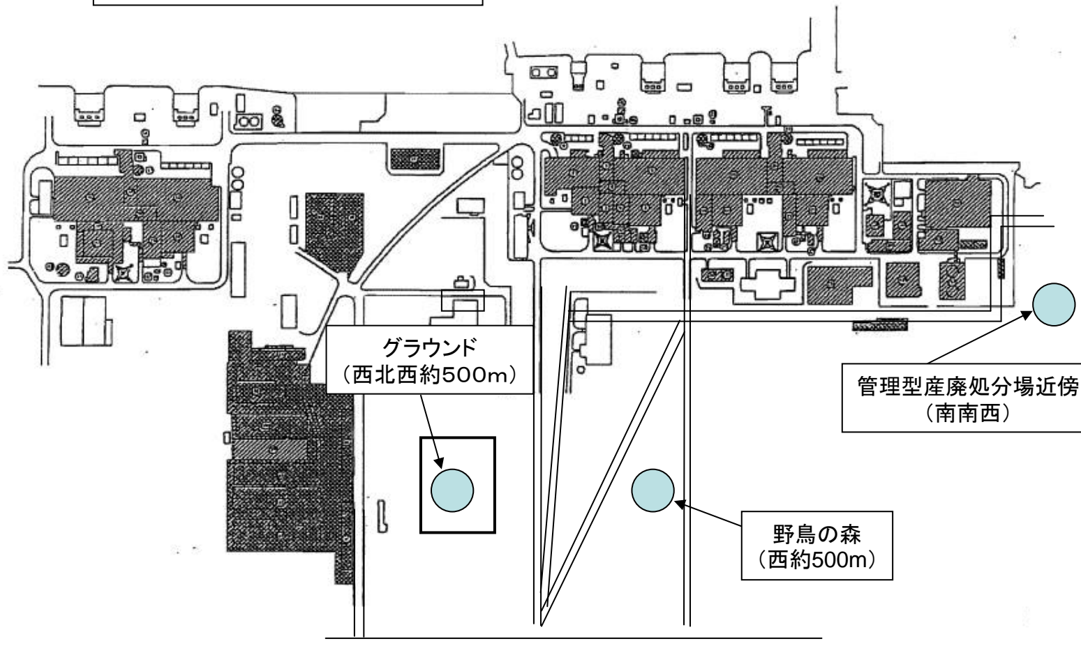
図面名称 福島第一原子力発電所 管理区域全体図
